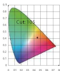
CIE 1931 x y Chromaticity Diagram
